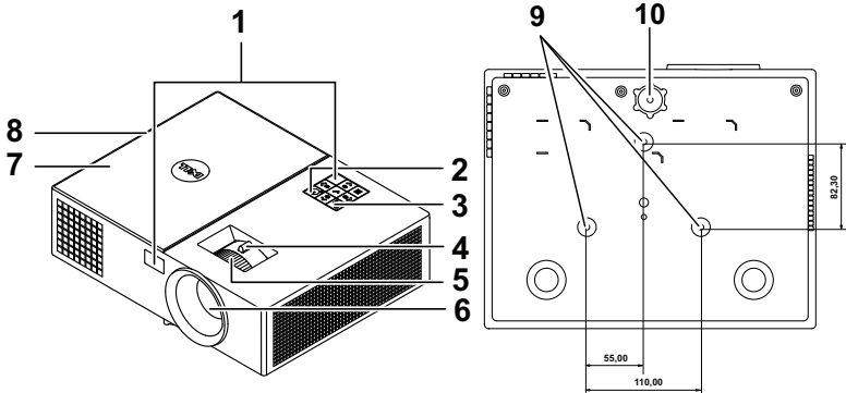
Vista Superior
